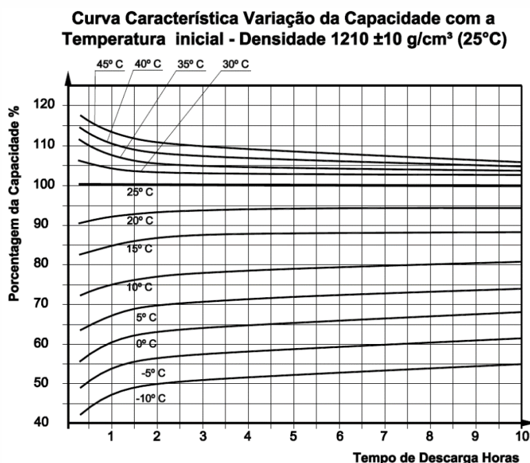
Fig.37 – Variação da Capacidade em função da temperatura do eletrólito
