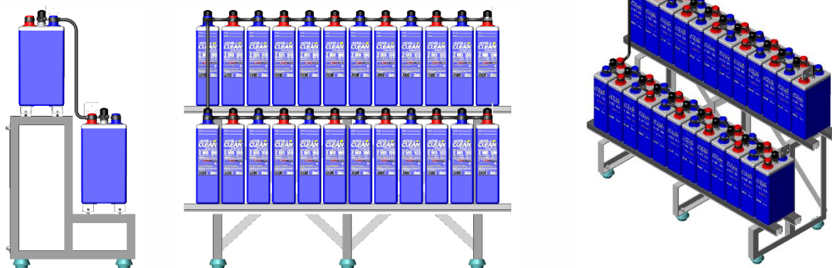
FIG.26- Exemplos de Montagem da Bateria (estante tipo degraus)
