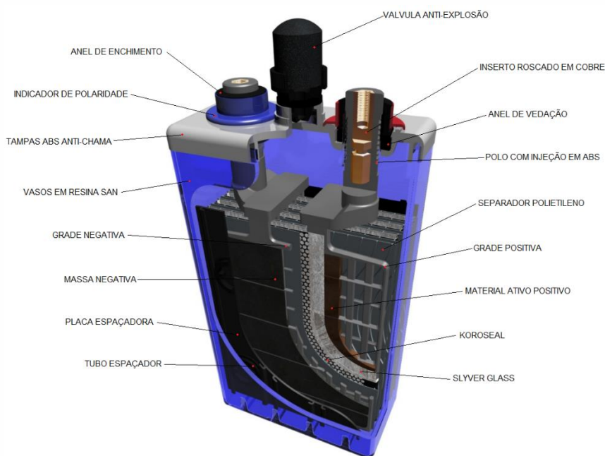
Fig.01- Características Construtivas Elemento 2V – Imagem Ilustrativa
