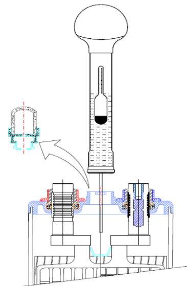
Fig.38 – Medição da Densidade - Ilustrativo
