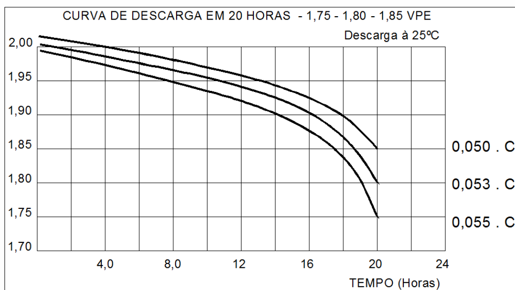
Fig.07 – Curva de descarga em 20 horas e Tensões finais de 1,75 – 1,80 e 1,85 VPE
