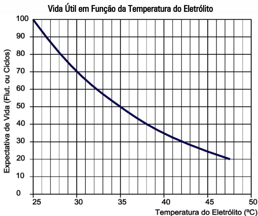
Fig.41– Curva de Redução da Vida útil x Temperatura do Eletrólito
