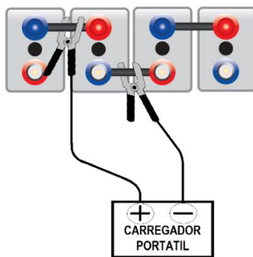
Fig.17 – Carregador Portátil para Carga Isolada.
