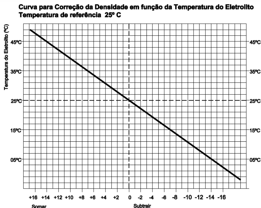
Fig.36 – Curva de Correção da densidade em função da temperatura do eletrólito
