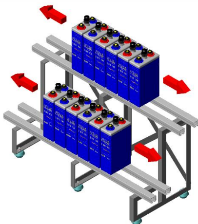
FIG.33- Instalação dos elementos na estante
