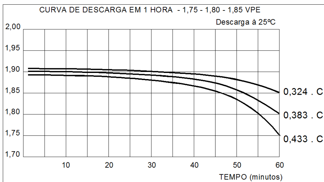
Fig.03 – Curva de descarga em 1 hora e Tensões finais de 1,75 – 1,80 e 1,85 VPE
