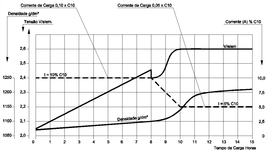
Curva Característica de Carga com Corrente Constante - "I" 0,10 e 0,05 x C10 - Dois Níveis
