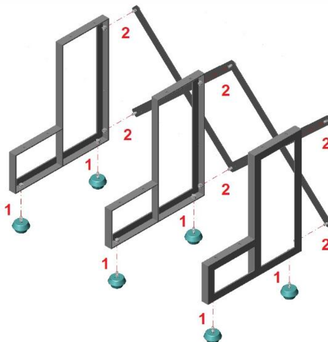
FIG.29- Quadros-Tirantes -Isoladores
