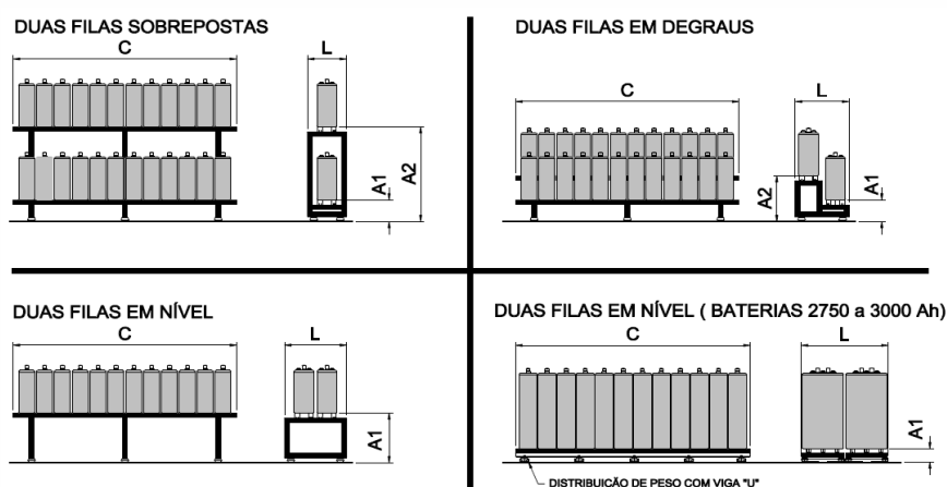
Fig.08 – Desenho de Estante Padrão e Detalhes Construtivos
