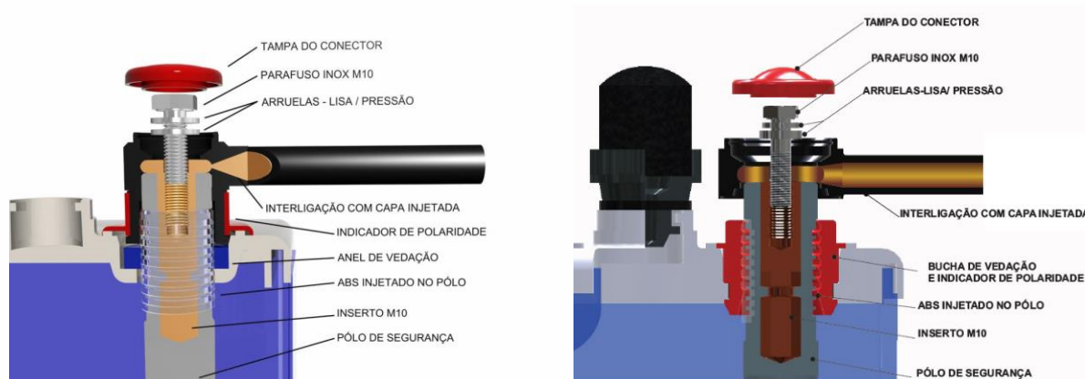
Fig.02 – Vedação Polo Tampa – Desenho Ilustrativo "A" e "B" bucha única de vedação
