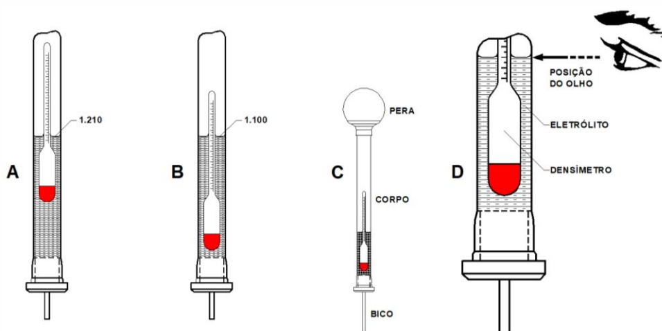
Fig.39 – Leitura da Densidade
