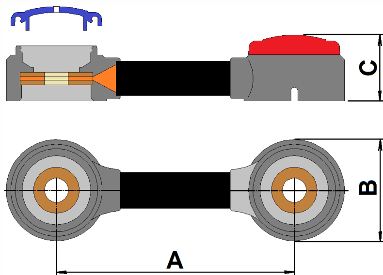
Fig.45. conector injetado
