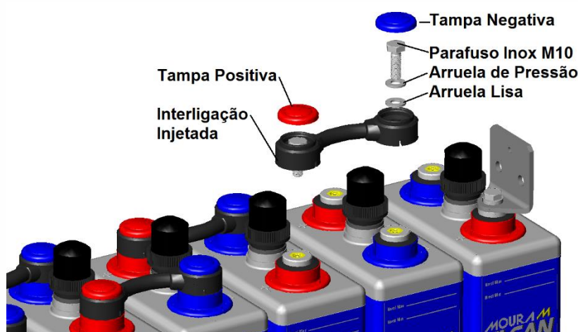
FIG.34- Instalação das conexões entre elementos
