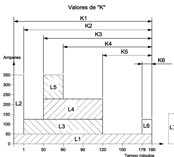
Fig. 42- Diagrama para distribuição das cargas
