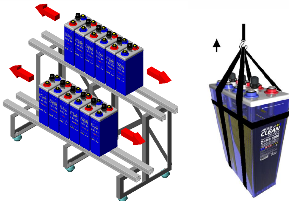
FIG.20- Instalação dos elementos na estante
