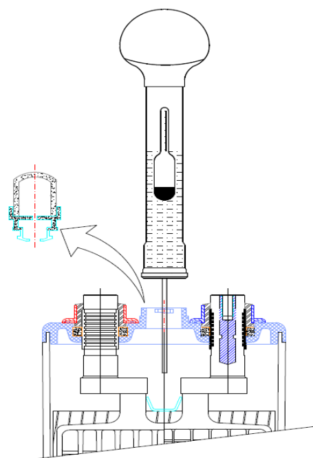
Fig.23 – Medição da Densidade – Ilustrativo
