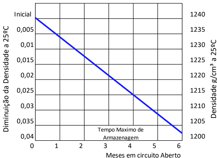
FIG.22- Densidade x Tempo
