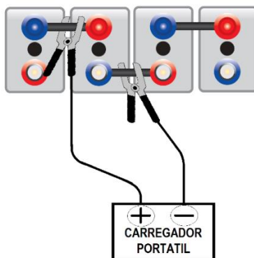
Fig.08 – Carregador Portátil para Carga Isolada.
