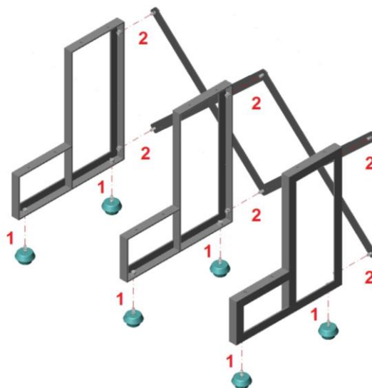
FIG.16- Quadros-Tirantes -soladores
