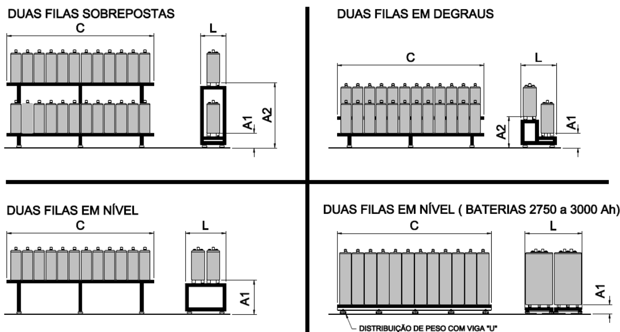
Fig.04 – Desenho de Estante Padrão e Detalhes Construtivos
