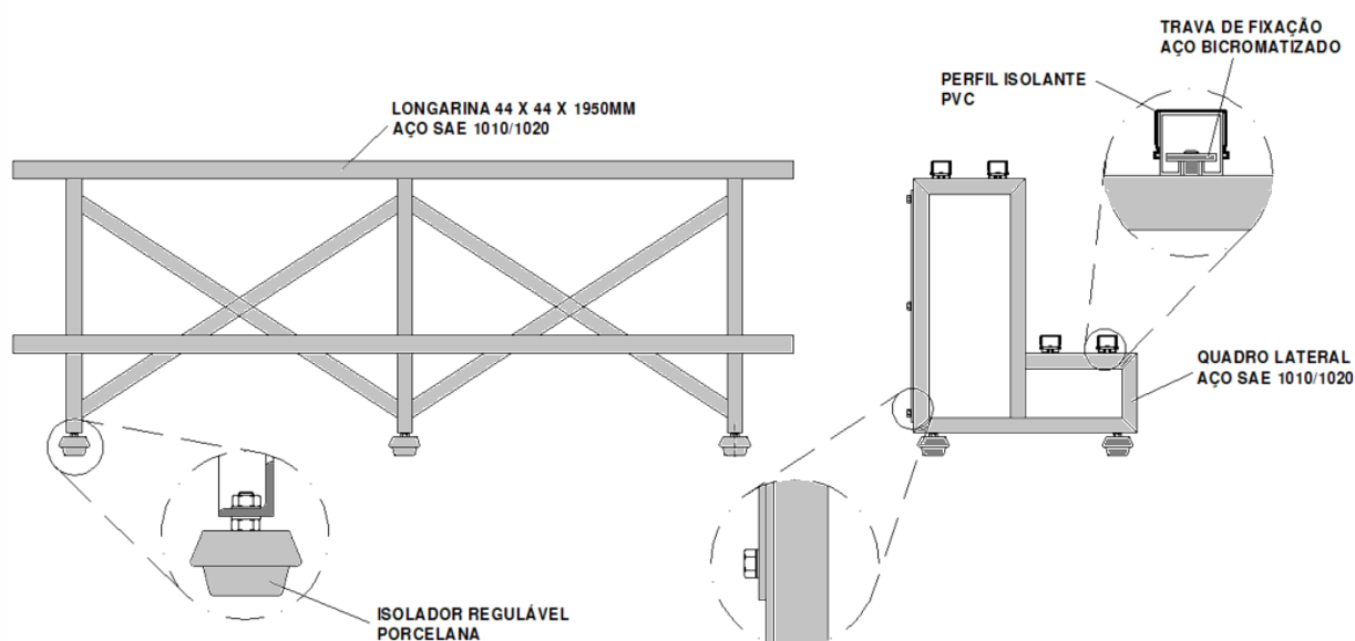
Fig. 03 – Exemplo de montagem, estante tipo degraus.
