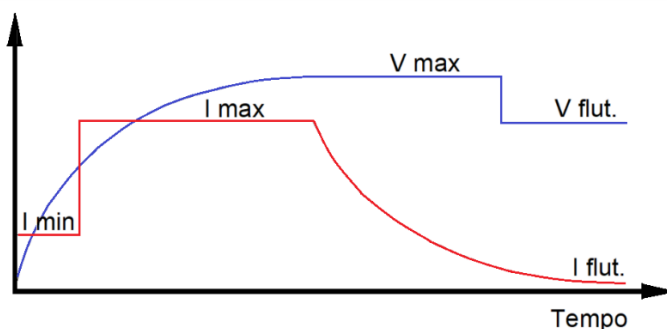
Fig.07 – Curva Característica de Recarga a 25°C
