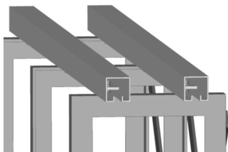
FIG.17- Fixação da Longarina
