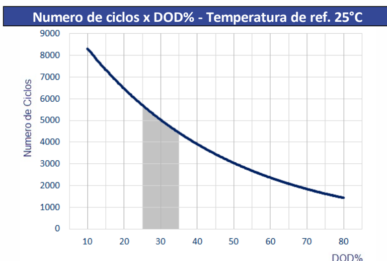
FIG.12- Característica de Vida em Ciclos a 25°C
