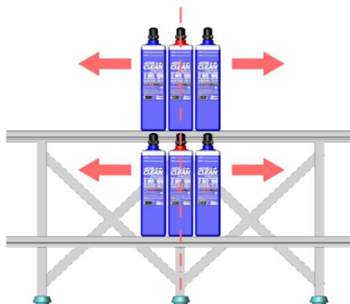
Centralização - número ímpar de elementos
