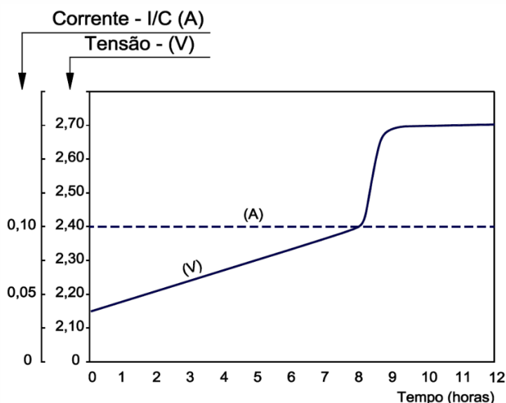
Fig.09 – Carga em Corrente Constante em um Nível
