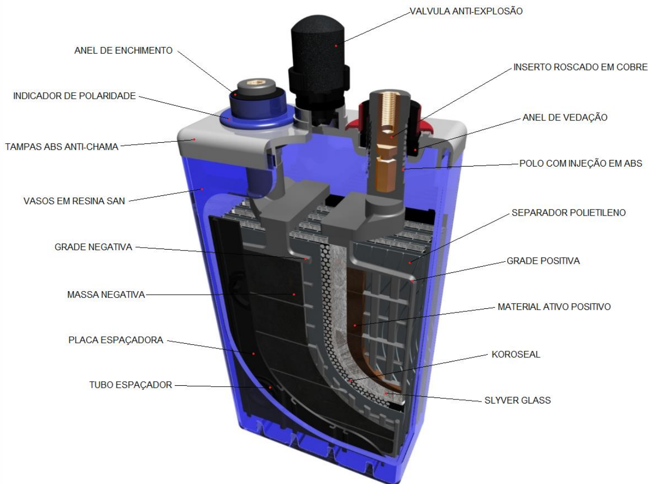
Fig.01- Características Construtivas – Desenho Ilustrativo
