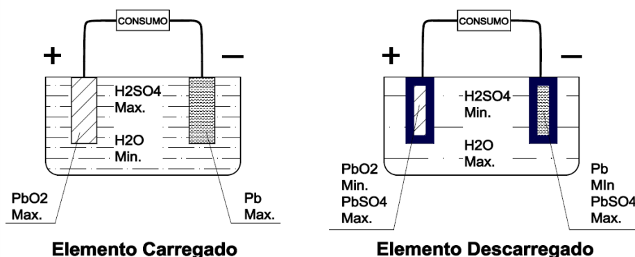
Fig. 11- Variações Qualitativas dos materiais ativos das placas positivas (+) e (-)
