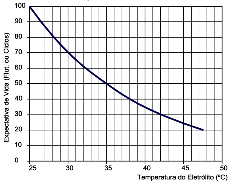
Fig.24 – Curva de Redução da Vida útil x Temperatura do Eletrólito
