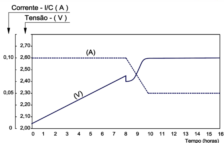
Fig.10 – Carga em Corrente Constante em dois Níveis
