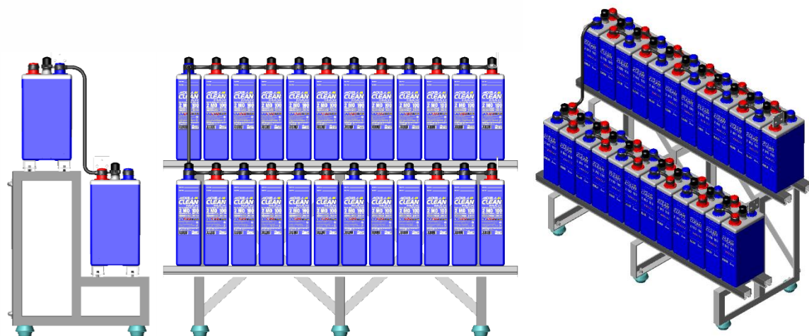
FIG.14- Exemplos de Montagem da Bateria (estante tipo degraus)
