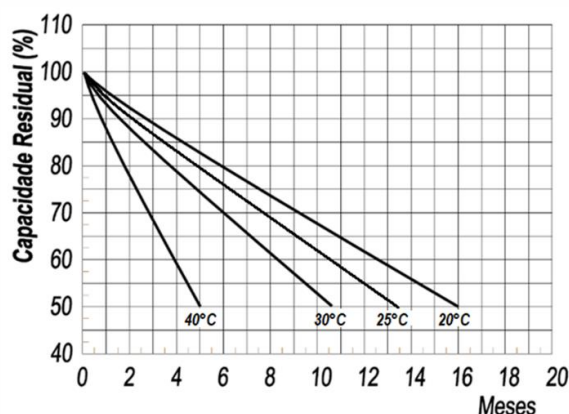
Fig.06 – Gráfico Ilustrativo da Auto Descarga x Tempo
