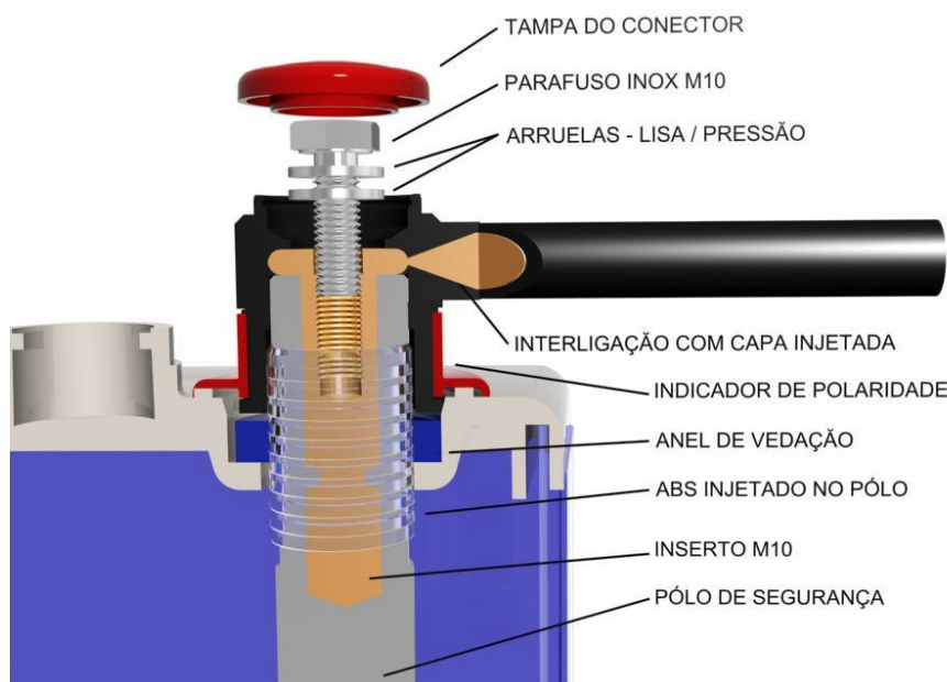
Fig.02 – Vedação Polo Tampa – Desenho Ilustrativo “A”
