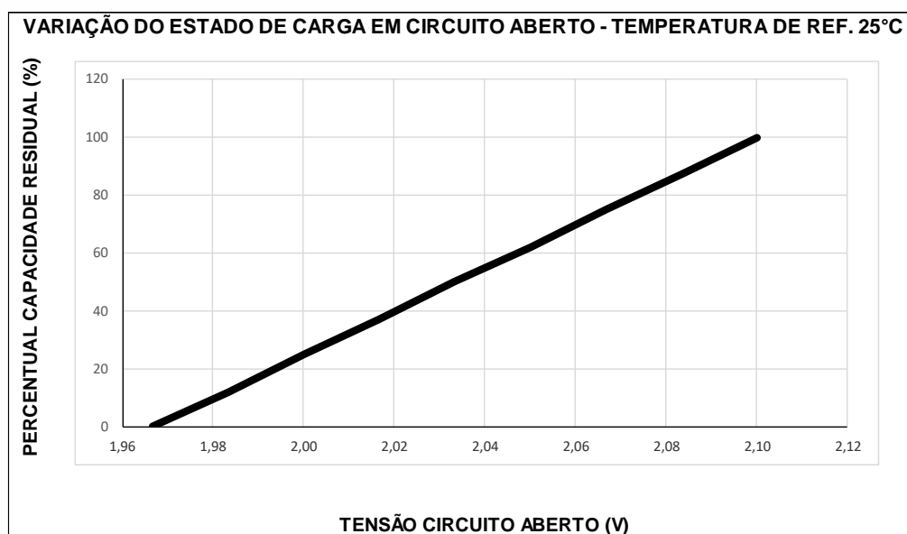
FIG.13- Característica de OCV x Capacidade
