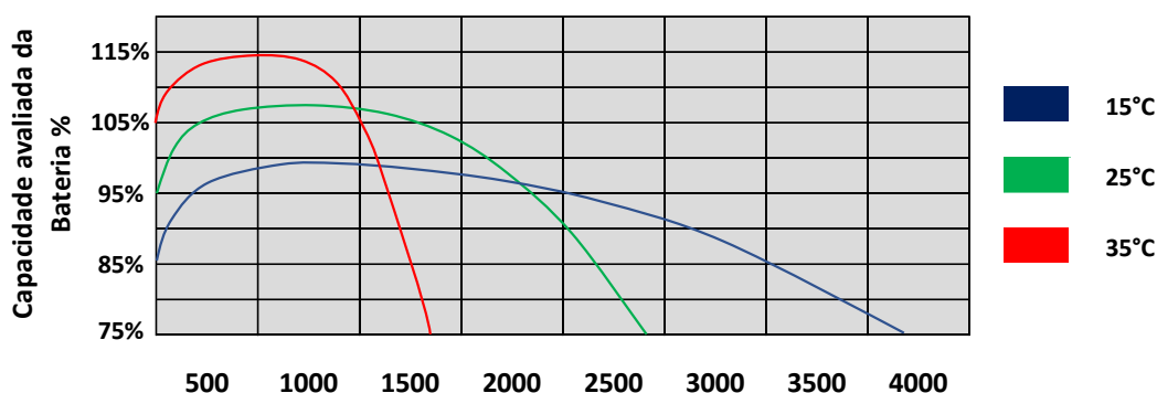
Fig.05 – Gráfico Ilustrativo Capacidade x Número ciclos para diferente temperatura
